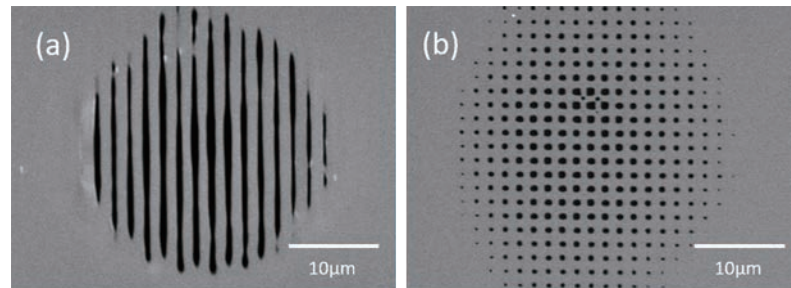
厚さが30 nmの支持基板のない薄膜をシングルショットレーザー干渉加工により作製した (a) 1次元格子と、(b) 2次元格子の例
