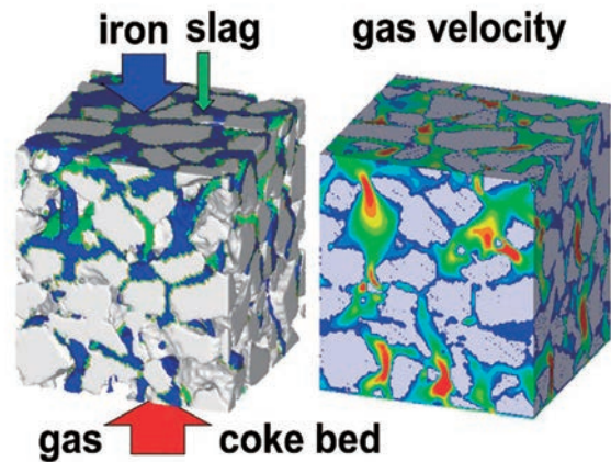
コークス充填層内の溶鉄・溶融スラグ・ガスの流動解析
