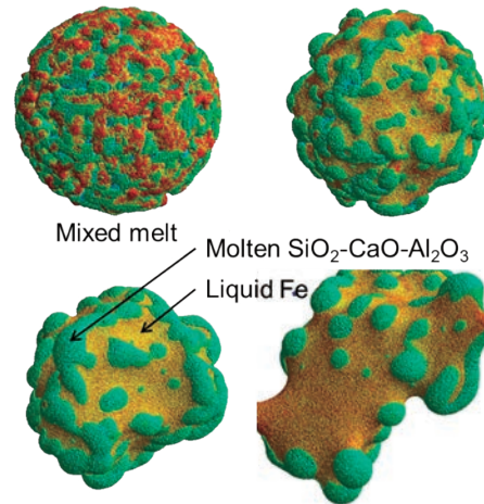
不混和二融体の分離過程
