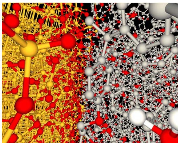
図 3. 分子動力学計算により得られたシリコン酸化膜（左）に接合するエポキシ主剤分子と硬化剤の原子・分子描像。
