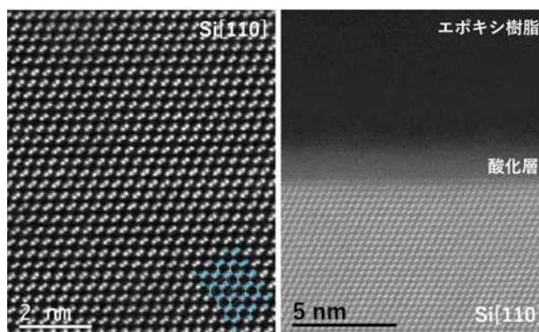
図 2. シリコン単結晶 (左図) およびシリコン単結晶基板とエポキシ樹脂の異種界面 (右図) の原子分解能電子顕微鏡像。
