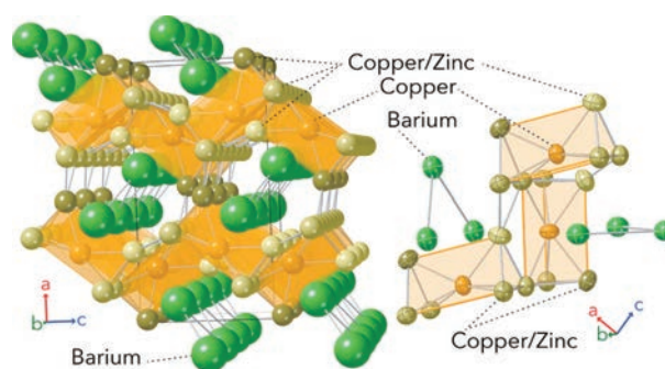
新規 \alpha -SrZn 5 型金属間化合物 BaCu 2.6 Zn 2.4 の結晶構造
