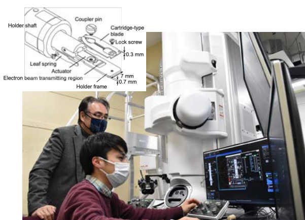
図 4. CREST 研究に使用する電子顕微鏡と試料延伸用特殊ホルダーの模式図（左上）。
