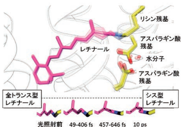
タンパク質 (バクテリオロドプシン) に含まれる発色団周辺の構造変化
