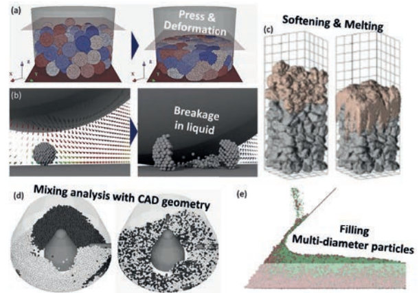
粉体現象および粉体プロセスのシミュレーションによる解析：(a) 圧縮成形時の粒子の変形挙動、(b) 湿式ボールミル中の粒子の運動・破壊挙動、(c) 鋳炉中の粒子の軟化溶融挙動、(d) CAD データを用いた粒子混合挙動、(e) 充填時の粒子偏析挙動
