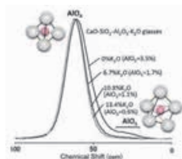
カルシウムアルミノケイ酸塩ガラスの 27 Al NMRスペクトルに及ぼす酸化カルウム添加の影響
