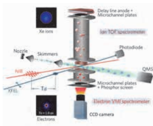
X線自由電子レーザーと超短パルスレーザーを組み合わせた実験装置
