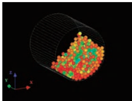
ロータリーキルン内の原料温度分布解析
