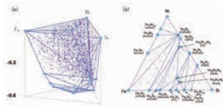
(a) 遺伝的アルゴリズムによって計算された Fe-Ni-Si 三元系基底状態における Convex-hull と (b) それを用いて構成した理論状態図。
