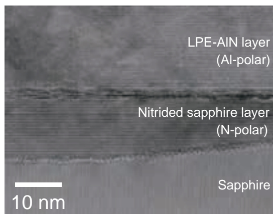
窒化サファイア基板上AIN膜の高分解断面TEM像
