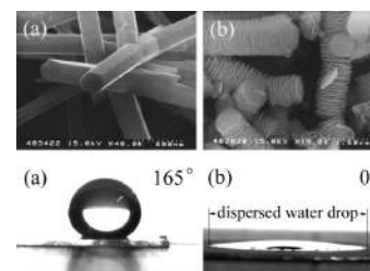
ソルボサーマル反応による超撥水性および超親水性ZnO薄膜の微細構造 Microstructure of superhydrophobic and superhydrophilic ZnO film prepared by the solvothermal reactions
