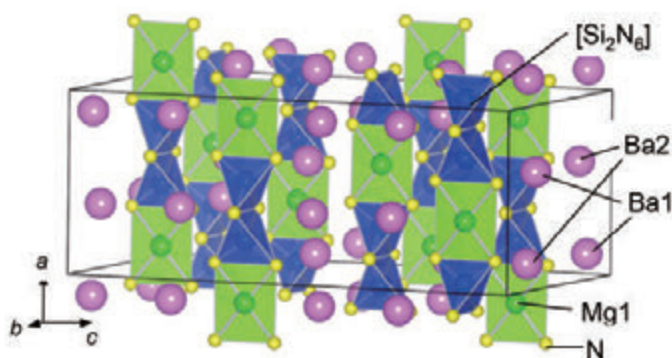
[Si 2 N 6 ] 10- の四面体二量体を含む 新規窒化物 MgBa 4 [Si 2 N 6 ] の結晶構造。 Mg 原子は N 原子により平面四配位されている
