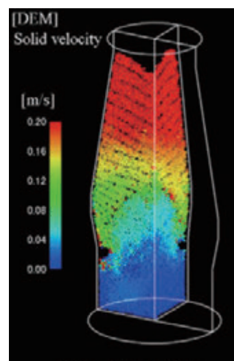
製鉄用高炉内の装入物降下挙動
