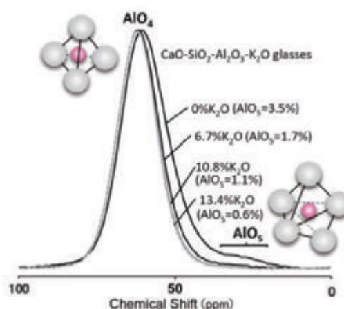
CaO-SiO 2 -Al 2 O 3 -K 2 O 系ガラス (K 2 O 添加量 = 0-13.4 mol%) の 27 Al MAS NMR スペクトル (18.8T)
