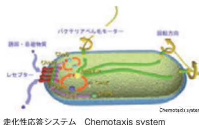
走化性応答システム Chemotaxis system
