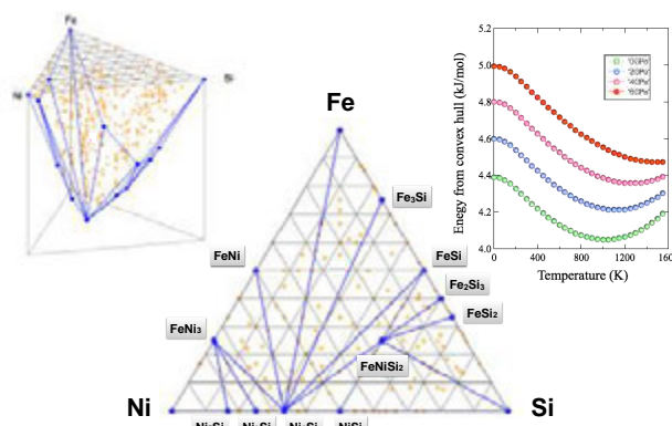
コンビナトリアル法を用いた合金系の安定構造の探索
