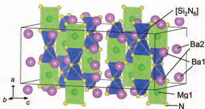
[Si 2 N 6 ] 10- の四面体二量体を含む 新規窒化物 MgBa 4 [Si 2 N 6 ] の結晶構造。 Mg 原子は N 原子により平面四配位されている
