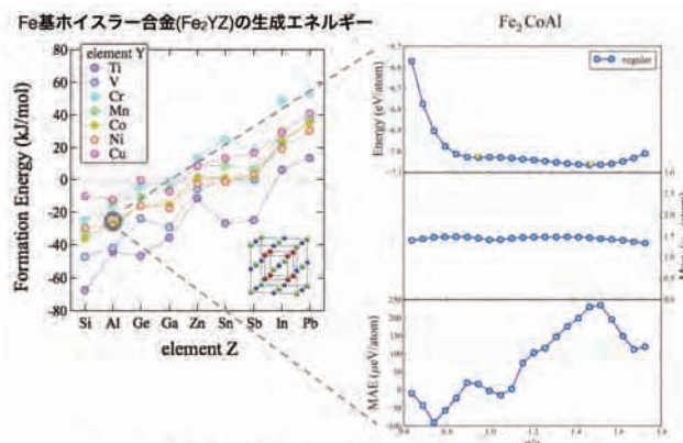
コンビナトリアル法による安定相・準安定相の探索
