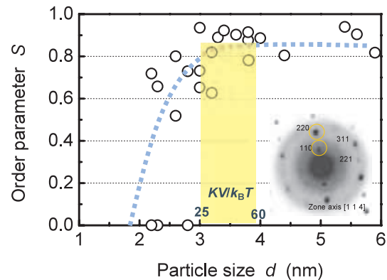
L1 0 FePt粒子の規則度の粒子サイズ依存性。K B T/k B Tは熱安定性指標。挿入図は一粒子からの電子回折パターン。
