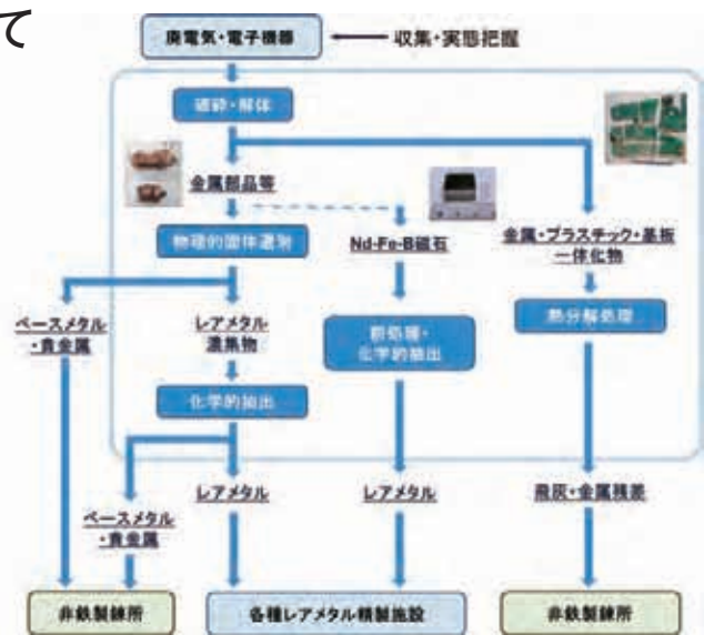
研究開発の範囲 (廃電気・電子機器からの希少元素精製)
