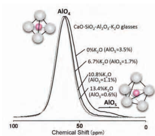
CaO-SiO 2 -Al 2 O 3 -K 2 O 系ガラス (K 2 O 添加量 = 0-13.4 mol%) の 27 Al MAS NMR スペクトル (18.8T)
