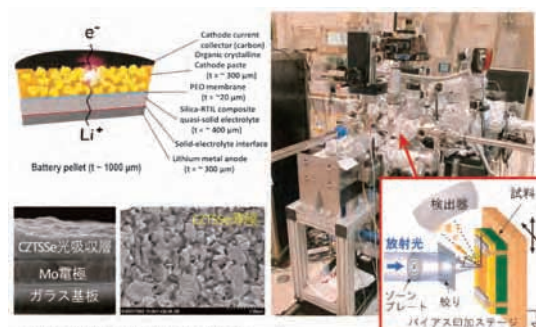
(上) 有機分子活物質を用いた全固体型リチウムイオン二次電池 (下) 超臨界流体プロセスで作製した化合物半導体薄膜太陽電池
