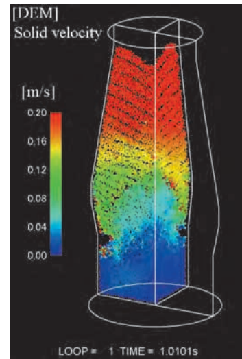
製鉄用高炉内の装入物降下挙動
