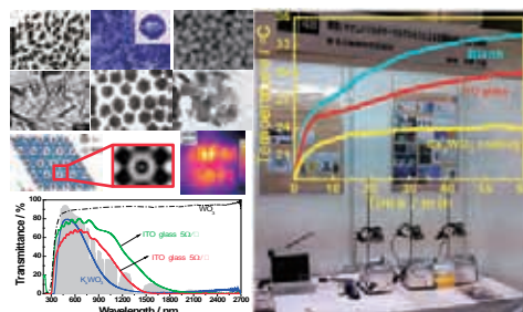
タングステンプロンの優れた熱線遮蔽特性 Excellent thermal shielding effect of the tungsten bronze.
