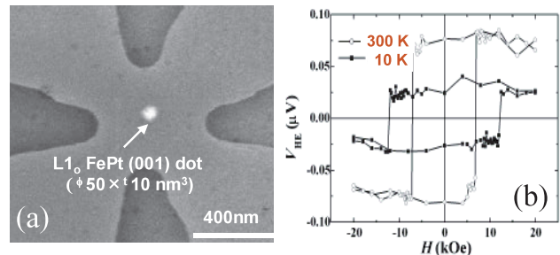
(a) L1 0 FePt (001)単結晶ドット測定用異常Hall効果測定デバイス, (b) 温度 T = 10, 300 Kにおける(a)のFePtドットの磁化曲線。
