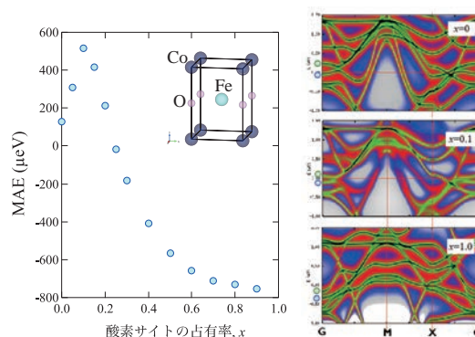
FeCoO x における垂直磁気異方性エネルギー(MAE)と電子バンドの酸素占有率依存性
