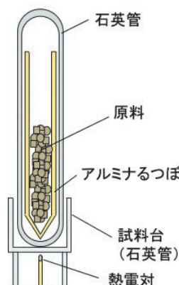
原料設置の概略図(左)およびブリッジマン炉(右)
