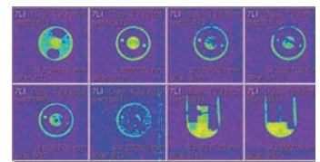
磁場勾配NMR装置とリチウム電池の 7 Liイメージング
