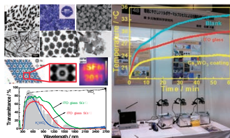
タングステンブロンズの優れた熱線遮蔽特性 Excellent thermal shielding effect of the tungsten bronze.
