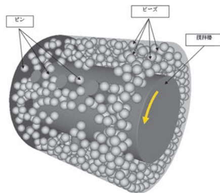
図2 媒体攪拌ミル内のビーズのDEMシミュレーションによる運動
