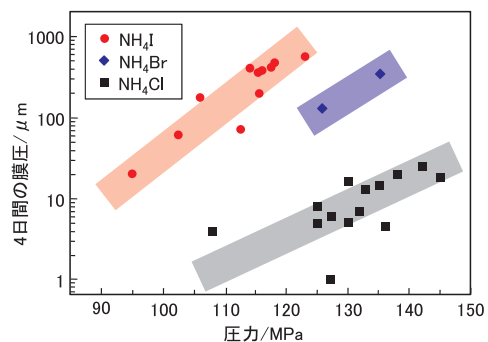
各鉱化剤NH 4 X(X=Cl, Br, I)における圧力と育成膜厚
