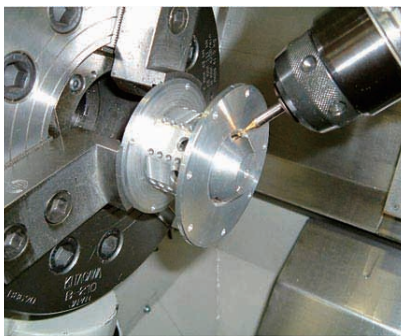
複合加工機による斜面への穴加工
