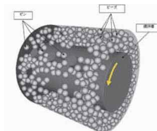
図2 媒体攪拌ミル内のピースのDEMシミュレーションによる運動
