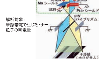
電子線ホログラフィーの 実験配置
