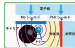
入射電子線を遮蔽するために、トナー粒子の上方にシールドを挿入。
