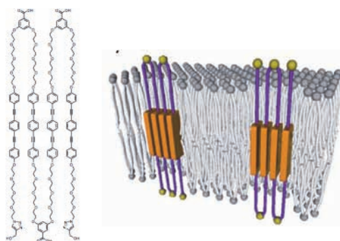
膜タンパク質を模倣したマルチブロック両親媒性分子
