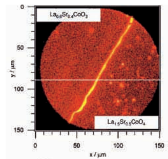
高性能空気電極を実現するナノヘテロ界面設計(明線が高速反応場)
