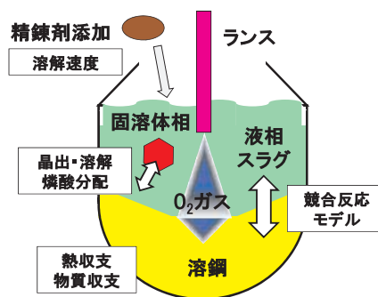
マルチフェーズスラグによる転炉精錬シミュレーションモデル
