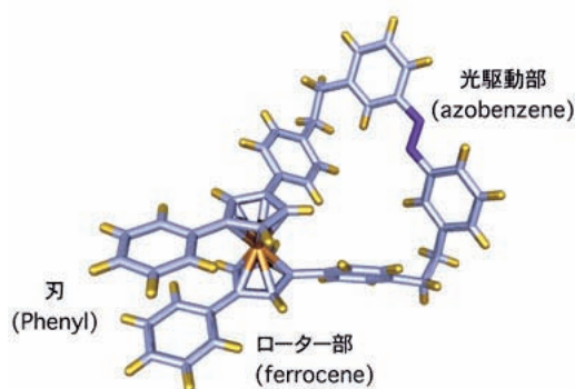
光に応答して開閉する光駆動分子はさみ
