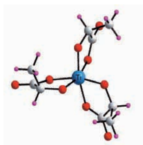
水溶性金属錯体
