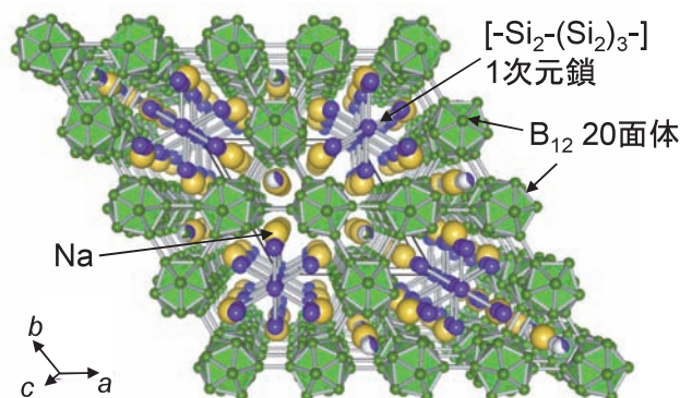
Na-B-Si系新規化合物 \text{Na}_8\text{B}_{74.5}\text{Si}_{17.5} の結晶構造
