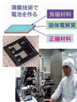
レーザー蒸着法で作成した薄膜リチウム電池
