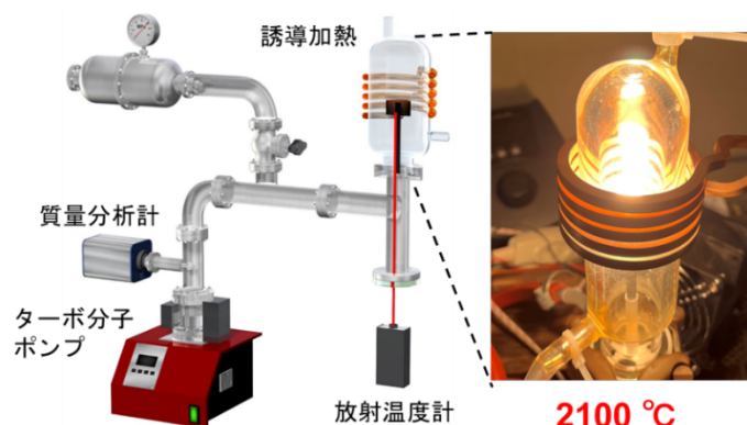
図 1. 超高温 TPD 装置の模式図
