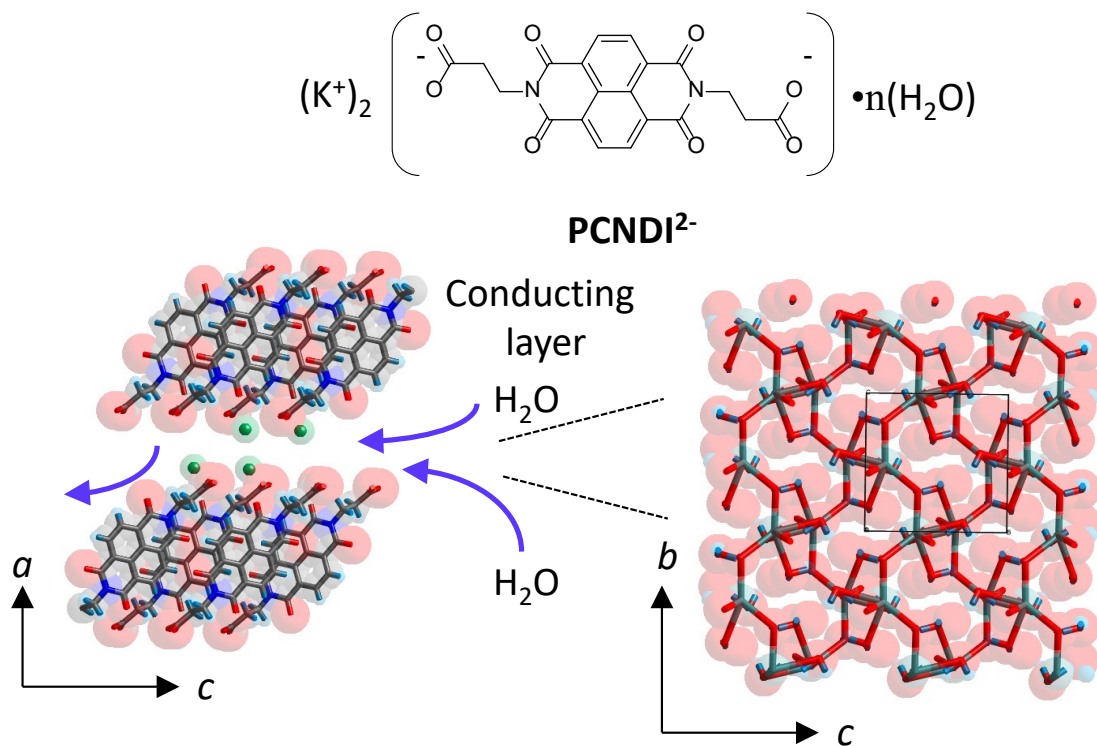
図 1 (K + ) 2 (PCNDI 2- )·n(H 2 O)の分子構造（上）と結晶構造（下）。結晶構造の b 軸投影図と PCNDI 2- が形成す二次元伝導層（左下）。伝導層間に存在するカチオン-アニオン静電ネットワークと水 H 2 O 分子の可逆的な吸脱着（左下）。
