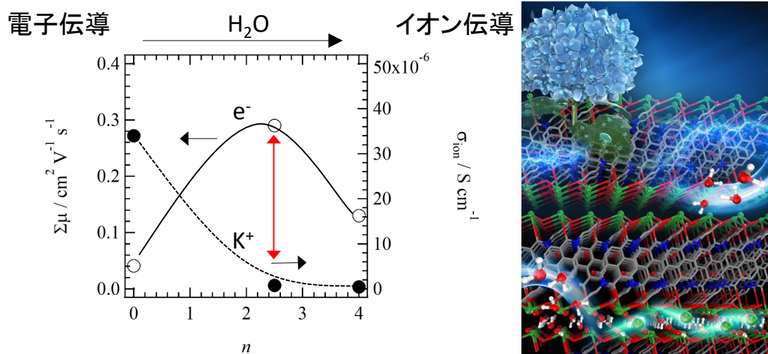
図 2 H 2 O 分子の二次元層に対する可逆な出し入れに伴う電子移動度（左軸）とイオン伝導性（右軸）の変化を示しています。水分量 n=2.5 の時に電子伝導性が最大になり、逆にイオン伝導性が最小となる事から、 n に依存した電子-イオン伝導スイッチングが観測されました。
