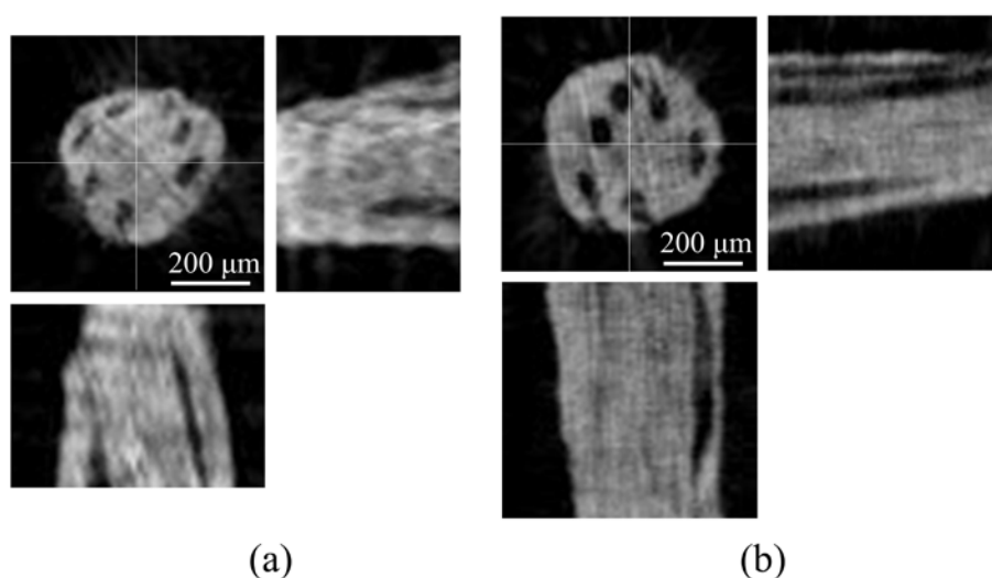
図 1 木片の CT 再構成結果。(a) Fourier 変換法の結果(露光時間 8.90 ms) [1]、(b) 縞走査法の結果(露光時間 4.43 ms)。
