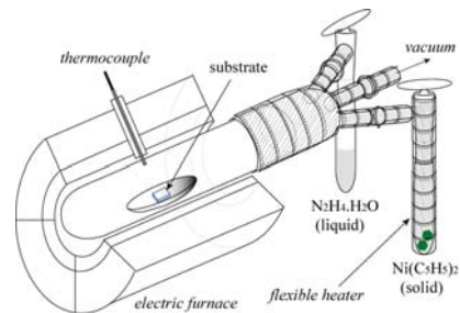
図1 CVRD実験装置図．
