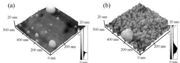
図2 無担時チタニア薄膜(a)とNiナノ粒子を担持した試料(b)のAFM図．
